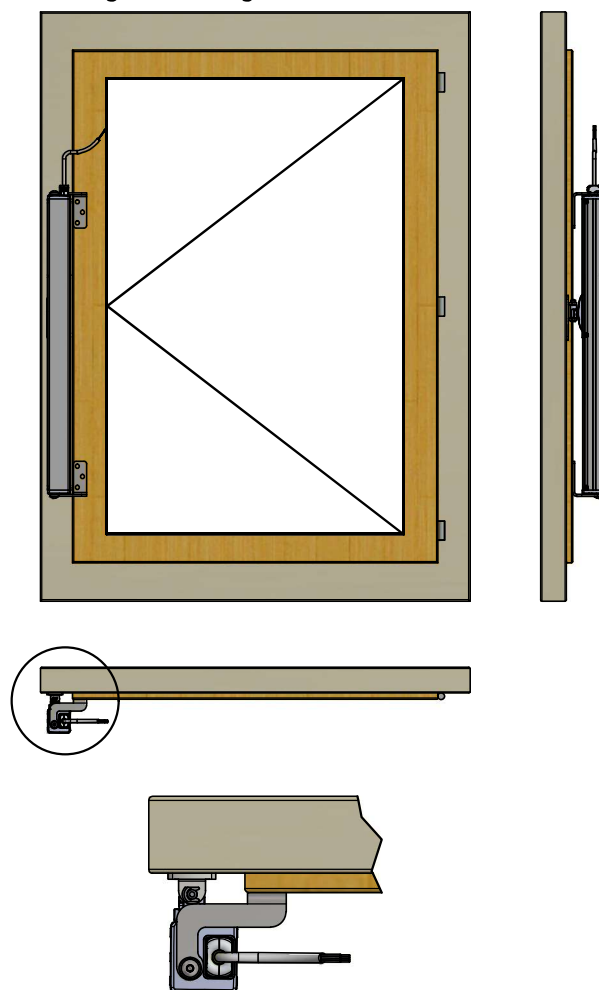
Abbildung 25: Am Flügel mitlaufend montiert
