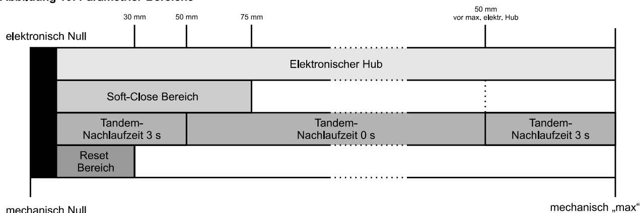
Abbildung 10: Parametrier-Bereiche
