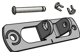
Abbildung 4: Obere Konsole K-K-OK-SK
