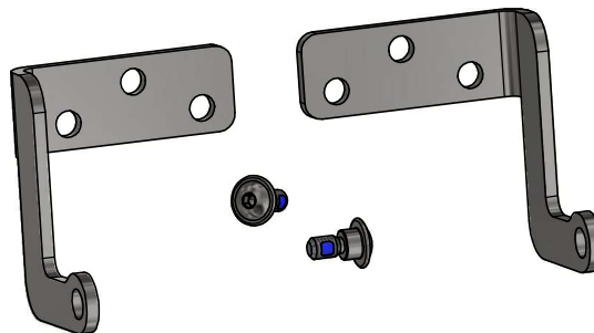
Abbildung 7: Untere Konsole K-K30-K
