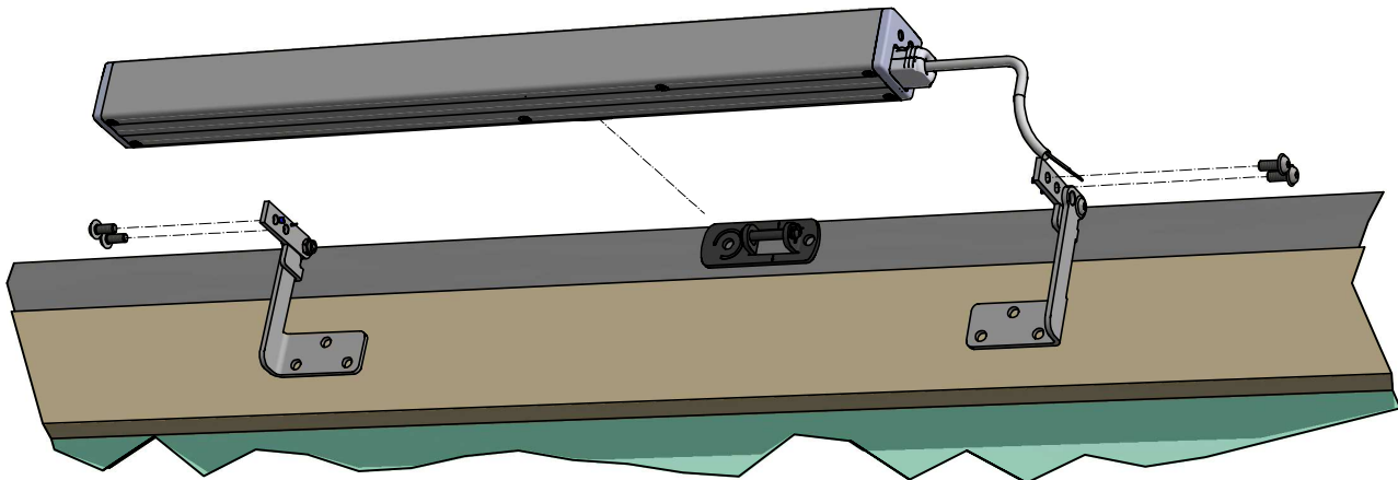
Abbildung 13: K-K30-FLEX
