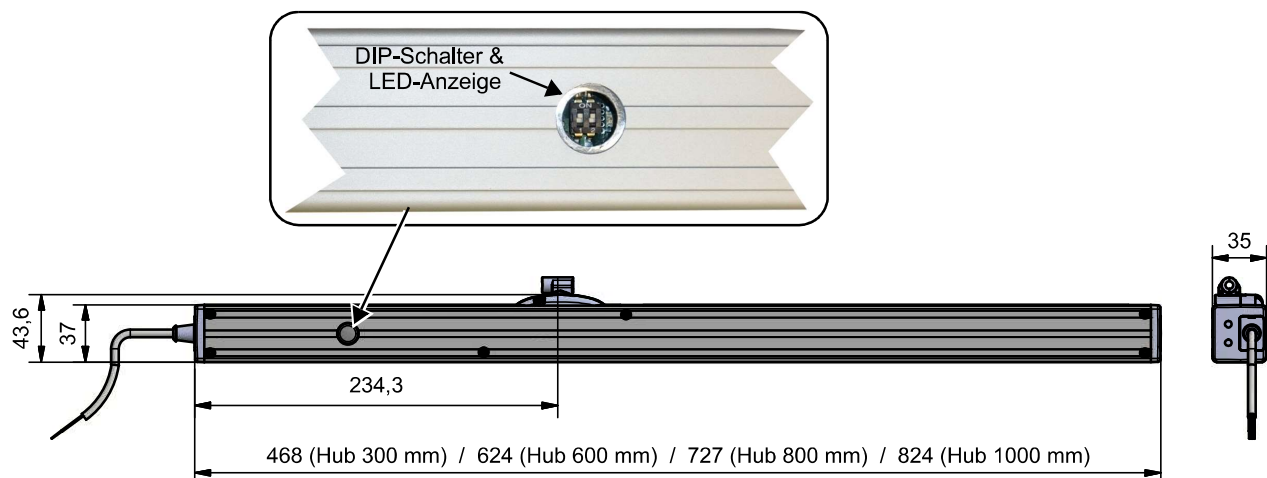
Abbildung 2: EA230-K-30/xxx(-S) Kettenantrieb
