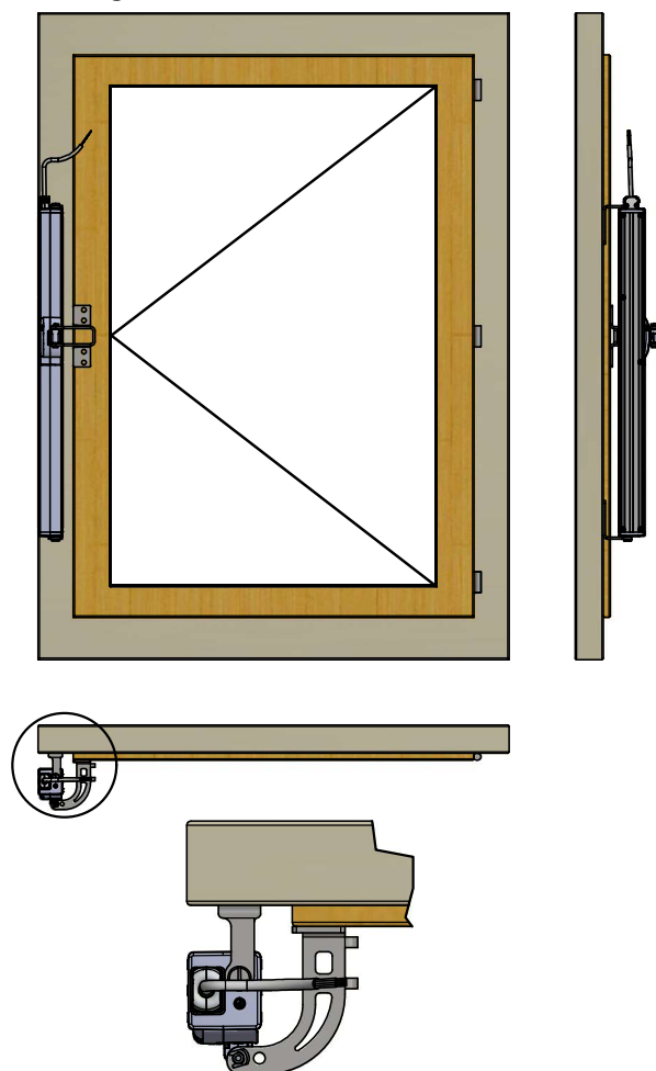
Abbildung 24: Am Blendrahmen montiert
