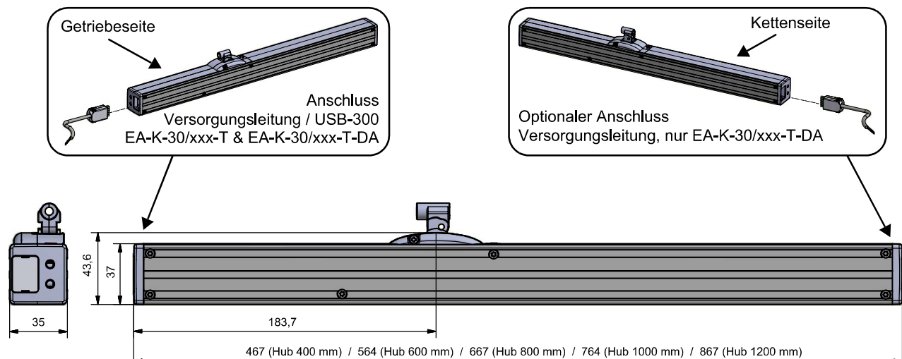
Abbildung 2: EA230-K-30/xxx(-S) Kettenantrieb
