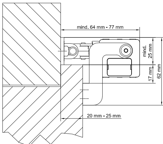
Abbildung 22: Kippflügel nach innen öffnend, mitlaufend
