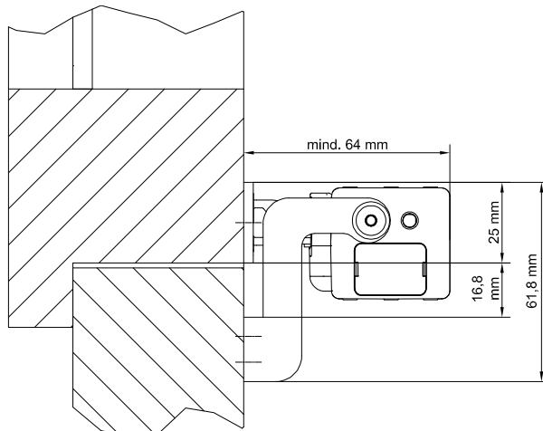
Abbildung 21: Klappflügel nach außen öffnend
