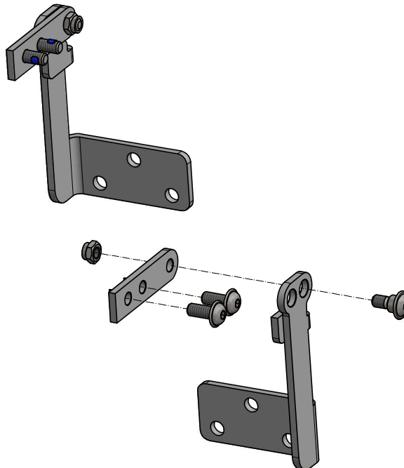
Abbildung 8: Untere Konsole – K-K30-FLEX
